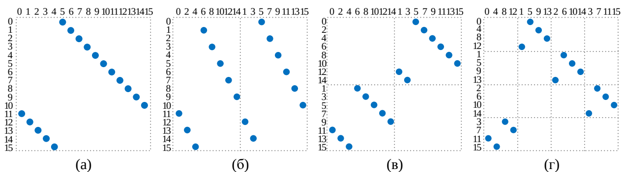
Слика 3.11. Примери дељења једног циркуланта на више мањих: (а) оригинални циркулант, (б) оригинални циркулант са пермутованим колонама за D = 2 , (в) финални пермутовани циркулант за D = 2 , и (г) финални пермутовани циркулант за D = 4 [58]
