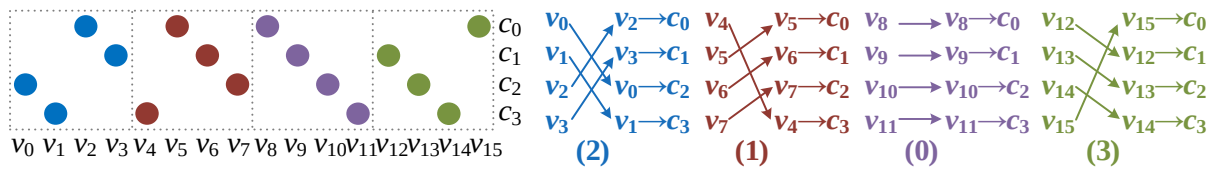
Слика 4.2. Пример једног слоја контролне матрице и одговарајуће потребне ротације у архитектури декодера за слојевито декодовање
