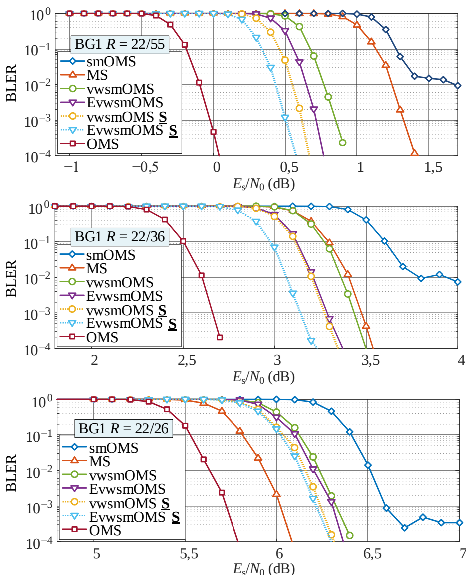
Слика 4.29. Перформансе различитих MS алгорита за кодове из 5G NR стандарда [60]
