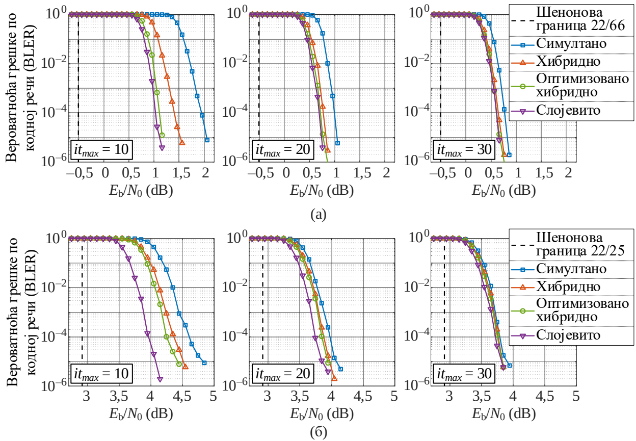
Слика 4.19. Перформансе контроле грешака за симултано, слојевито, хибридно и оптимизовано хибридно декодовање за кодове из 5G NR стандарда: (а) (25344, 8448) кодног количника R = 22/66 и (б) (9600, 8448) кодног количника R = 22/25 [49]
