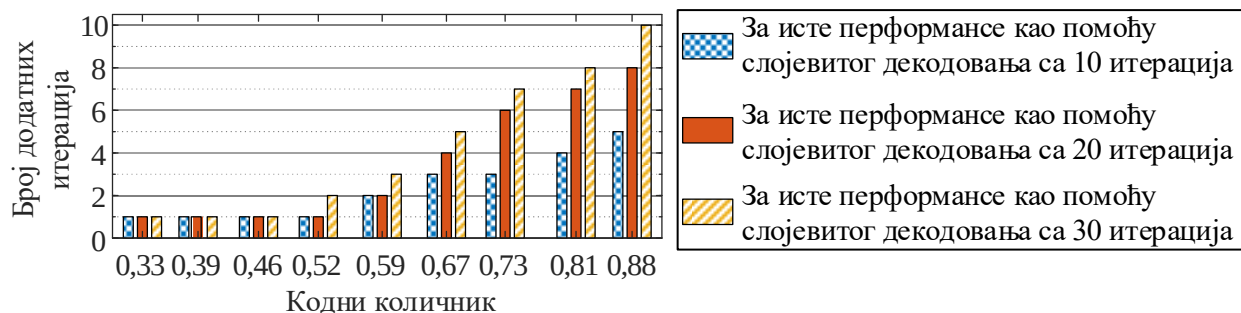
Слика 4.21. Потребан број додатних итерација оптимизованог хибридног декодера за исте перформансе контроле грешака као код слојевитог декодовања (исто E_b/N_0 за BLER 10^{-5} ) [49]
