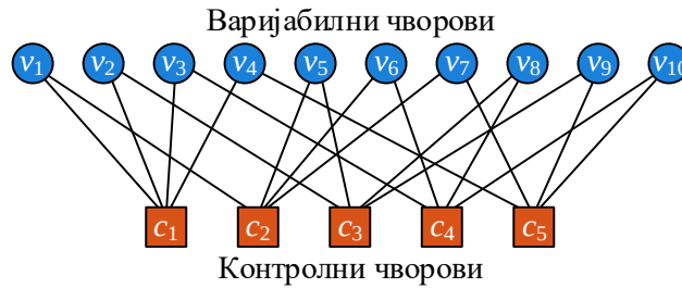
Слика 2.2. Представа LDPC кода помоћу Танеровог графа
