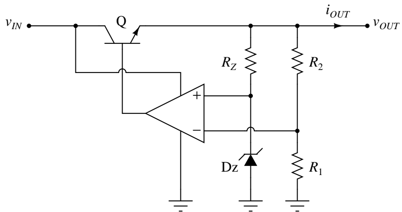
Slika 2: Stabilizator napona sa povratnom spregom, izvor referentnog napona na stabilisanoj strani.
