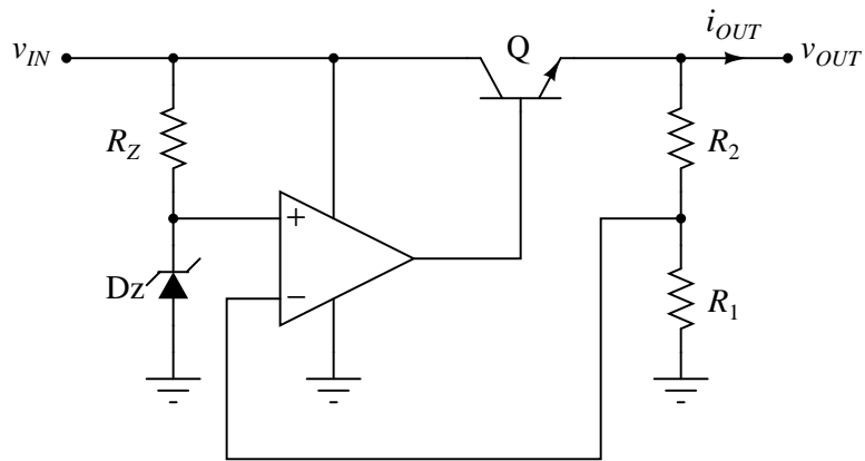
Slika 1: Stabilizator napona sa povratnom spregom.
