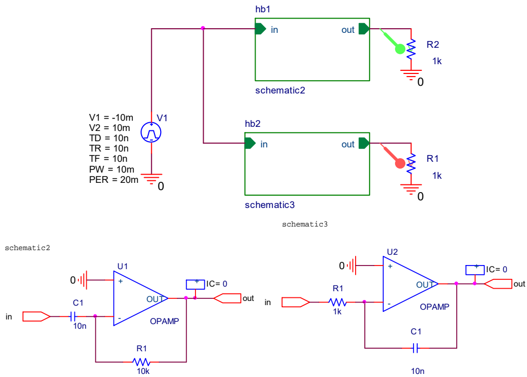
1. Hijerarhijski blokovi, diferencijator i integrator
