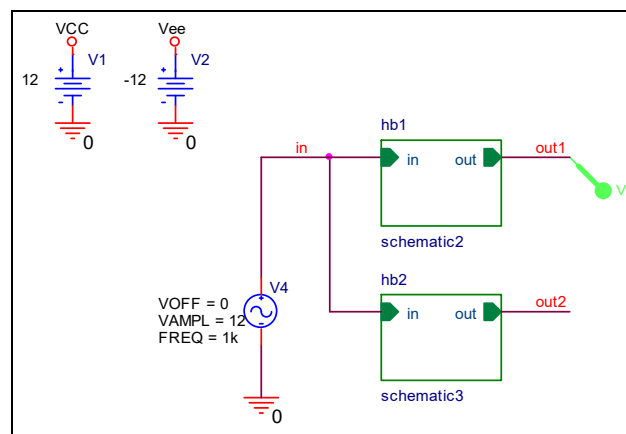
2. Hijerarhijski blokovi - komparatori sa histerezisom
